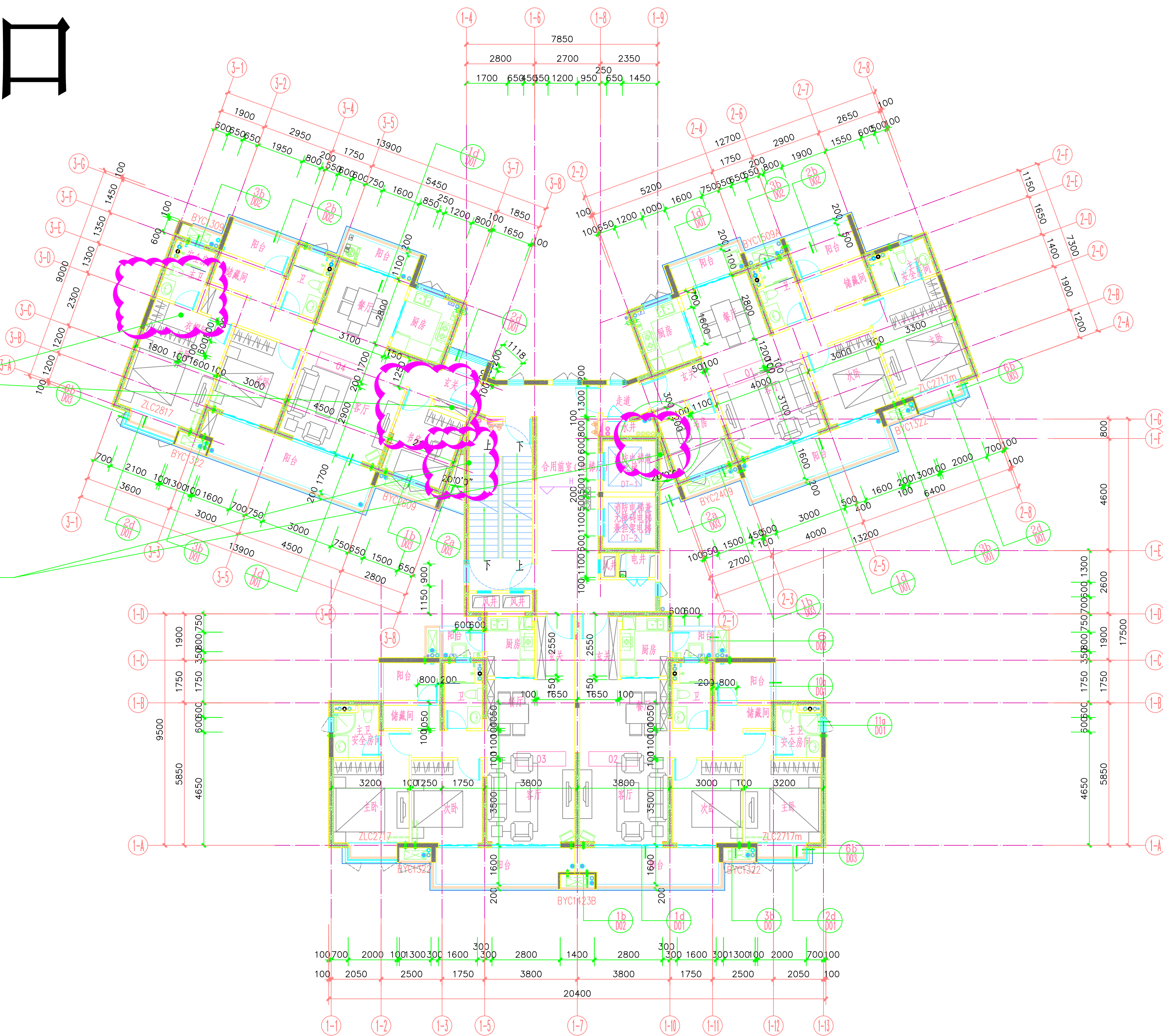
四~三十三层平面图 1:100
