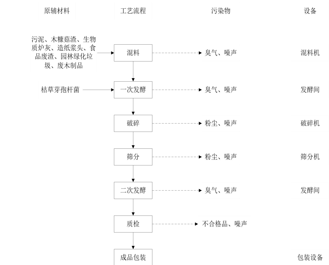
图 2-3 营养土生产工艺流程及产污环节图
