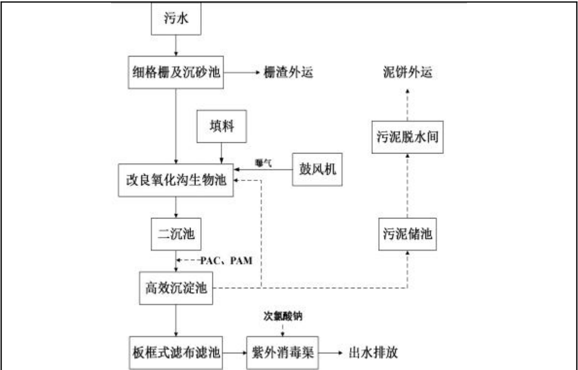
图 4-1 恩平产业转移工业园污水处理厂工艺流程图
