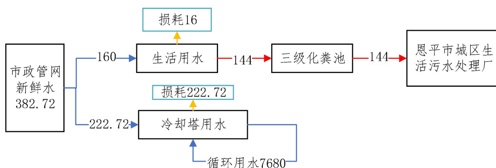
图2 项目水平衡图 (单位: m³/a)
