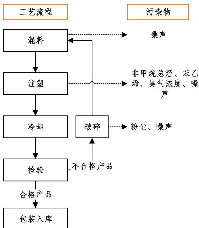
图2 项目产品生产工艺流程及产污过程图
