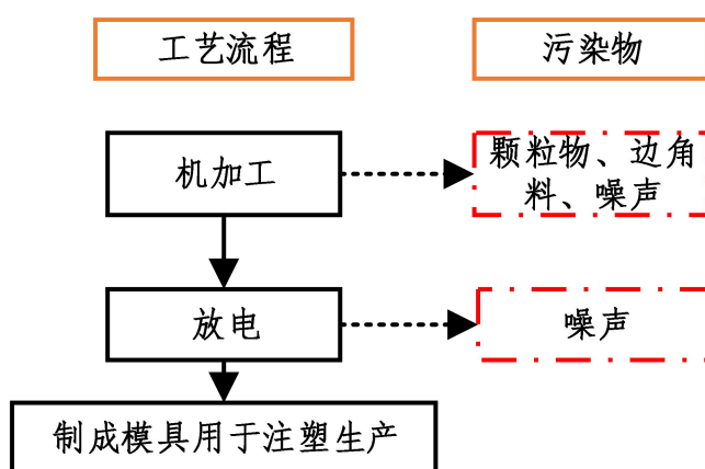
图1 项目配套模具生产工艺流程及产污过程图
